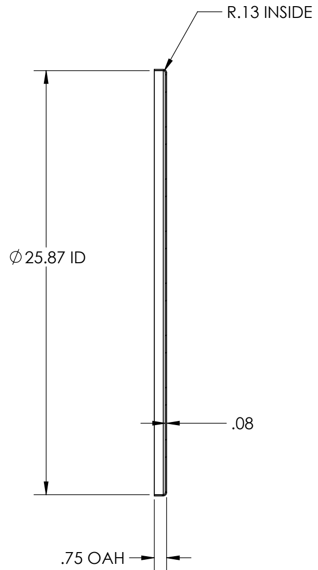
SECTION A-A SCALE 1 : 6
